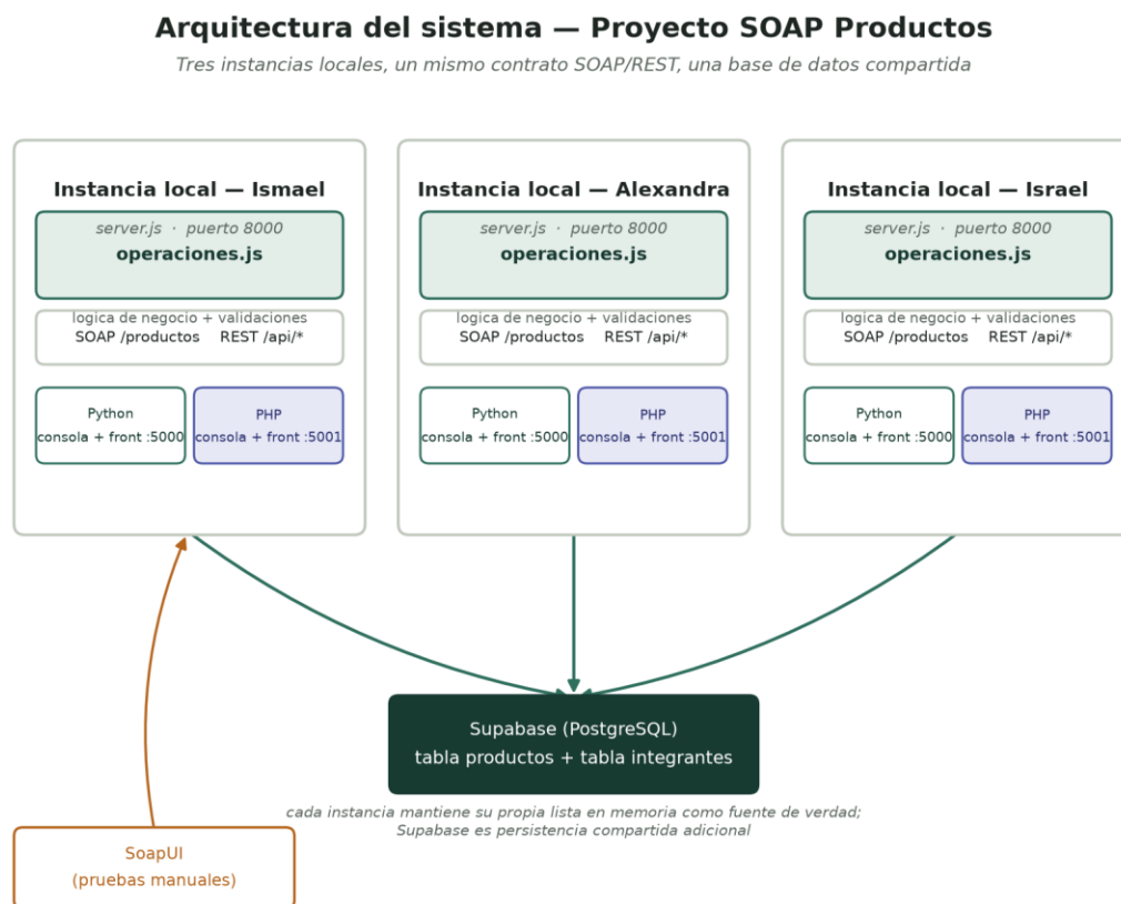
Figura 1. Arquitectura general del sistema: tres instancias locales, un mismo contrato SOAP/REST, una base de datos compartida.
