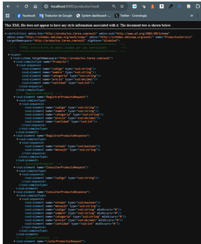
Figura 9. El documento WSDL completo, accesible directamente desde el navegador.
