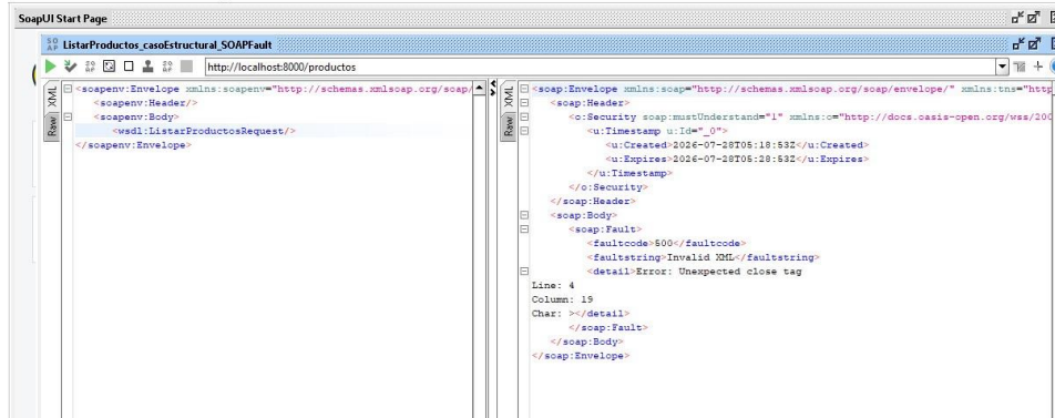
Figura 6. Como ListarProductos no recibe parámetros, se documentó en su lugar un XML mal formado para mostrar cómo el motor SOAP responde con un Fault ante una solicitud inválida en su estructura.
