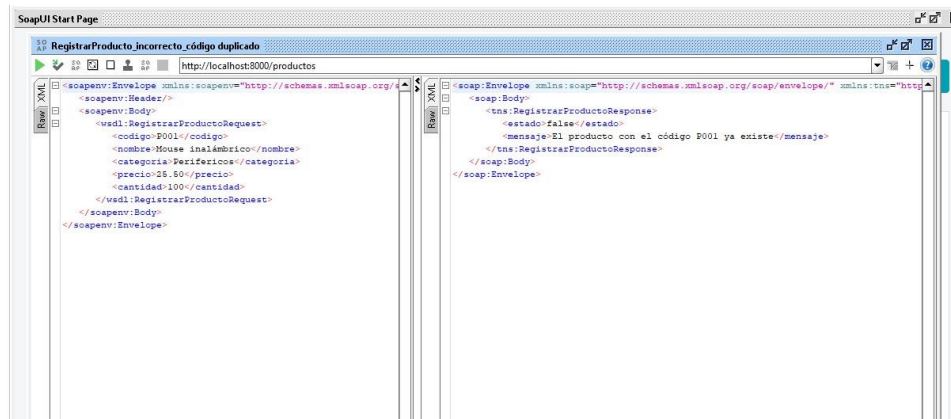
Figura 4. El servidor rechaza un código ya existente, devolviendo estado = false y un mensaje explicando el motivo.
