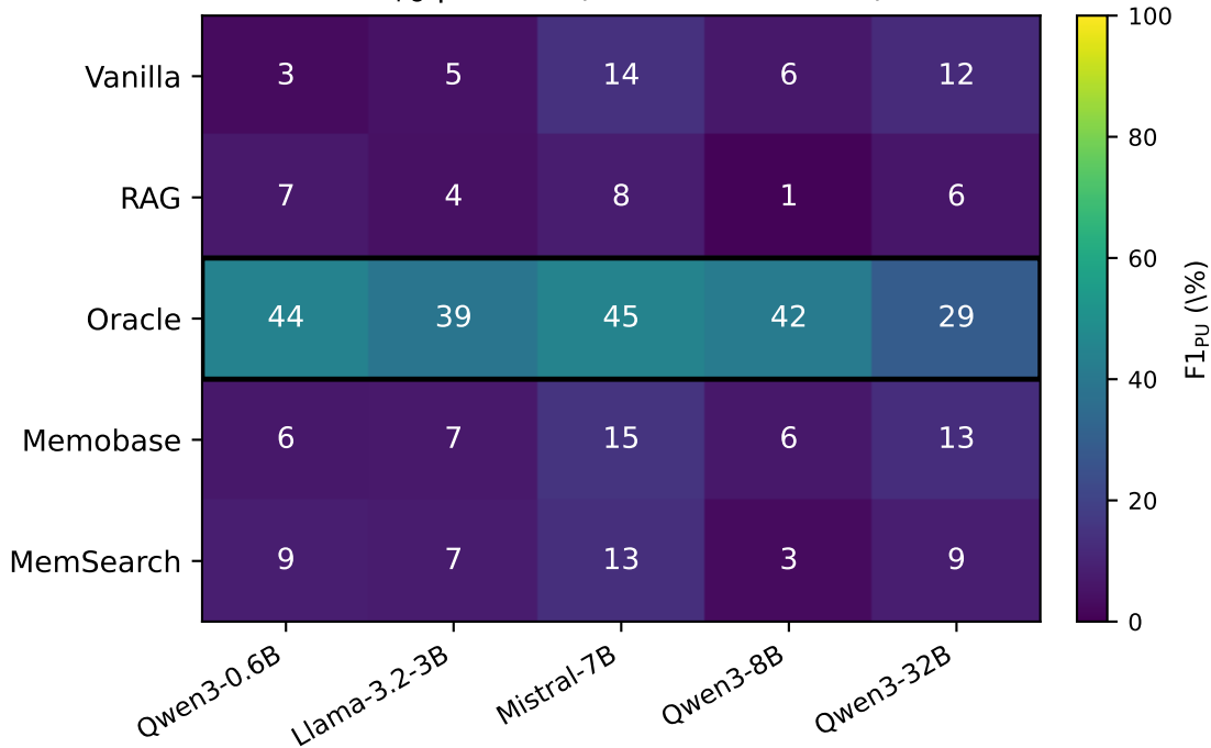
F1 PU per cell (Oracle row boxed)
