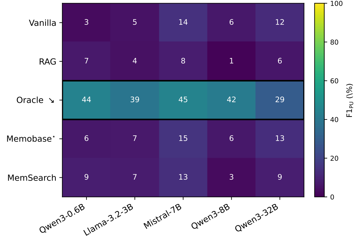
(c) F1 PU
