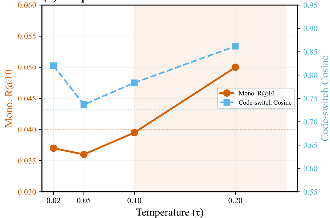
(d) Temperature Ablation: Retrieval & Code-switch
