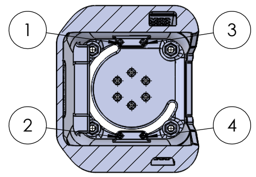
SECTION A-A SCALE 1 : 4
