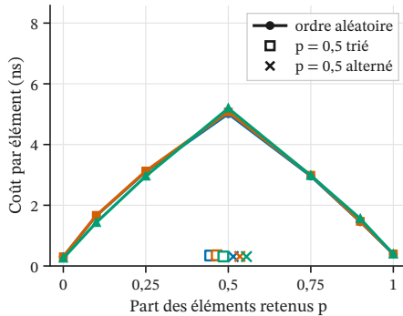
(e) Clang : filter_copy (if)
