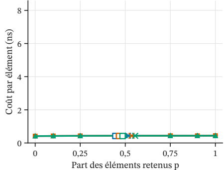
(f) Clang : filter_copy_mask
