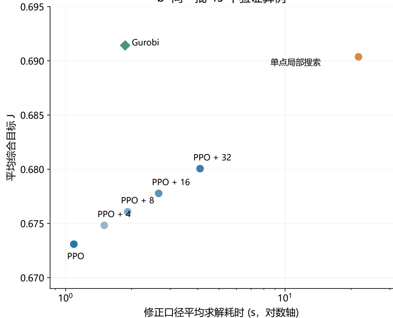
b 同一批 45 个验证算例
