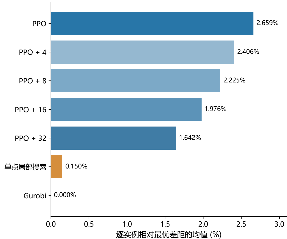
a 解质量相对精确最优的差距
