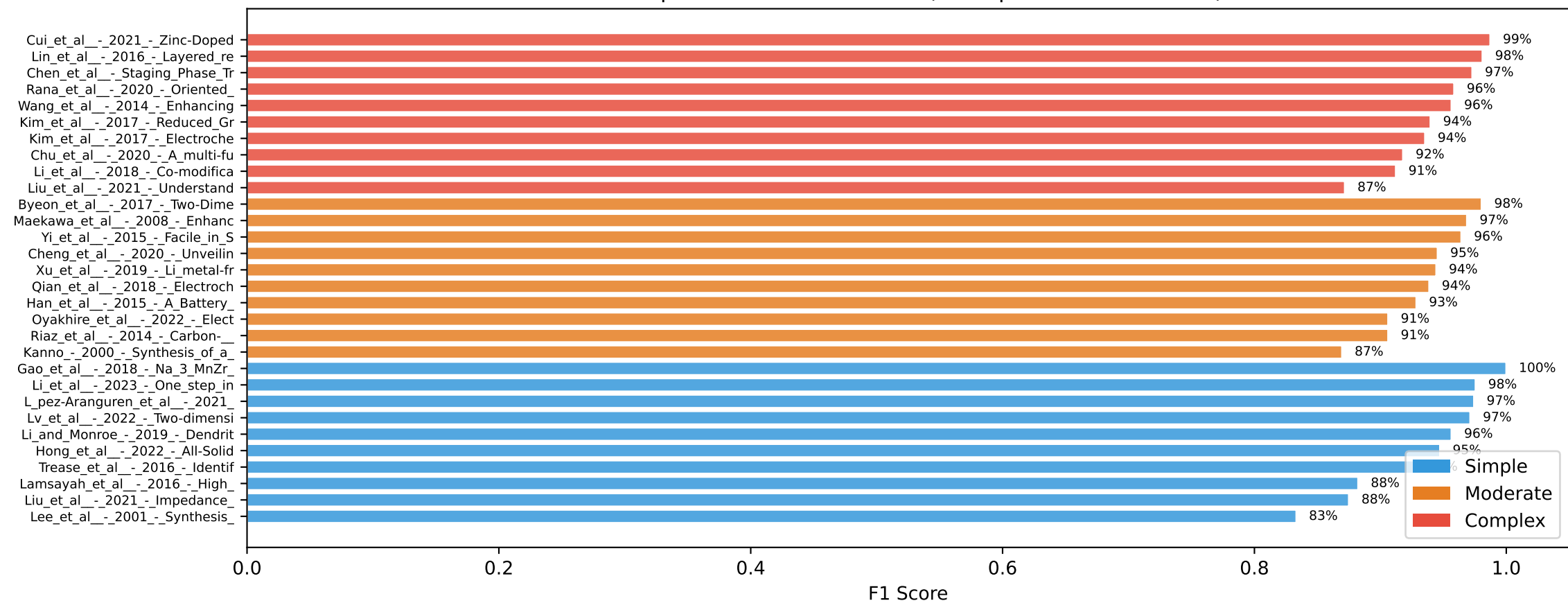
Per-Paper Extraction F1 Score (30-Paper Golden Dataset)
