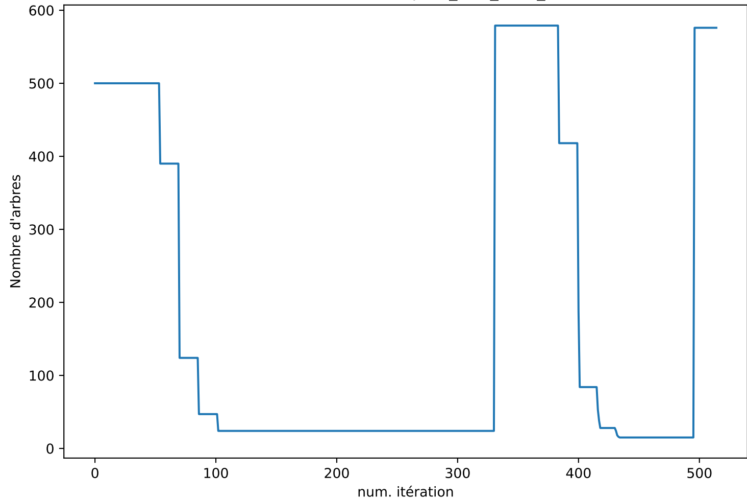
Nombre d'arbres au cours des itérations (prob_tree_after_rain=0.1 (default 0.02))
