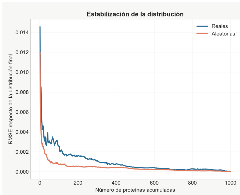
Figura 2: RMSE de la distribución acumulada respecto de la distribución final. La curva se estabiliza alrededor de las 500 proteínas.
