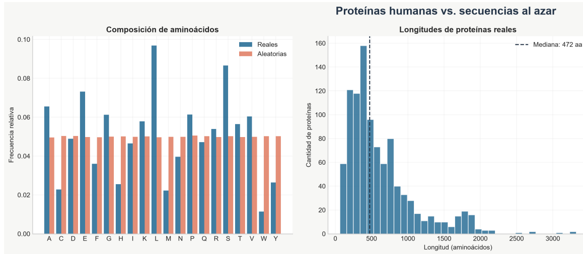
Figura 1: Distribución de aminoácidos de proteínas reales y aleatorias. Las proteínas reales muestran una composición no uniforme, a diferencia del modelo aleatorio equiprobable.
