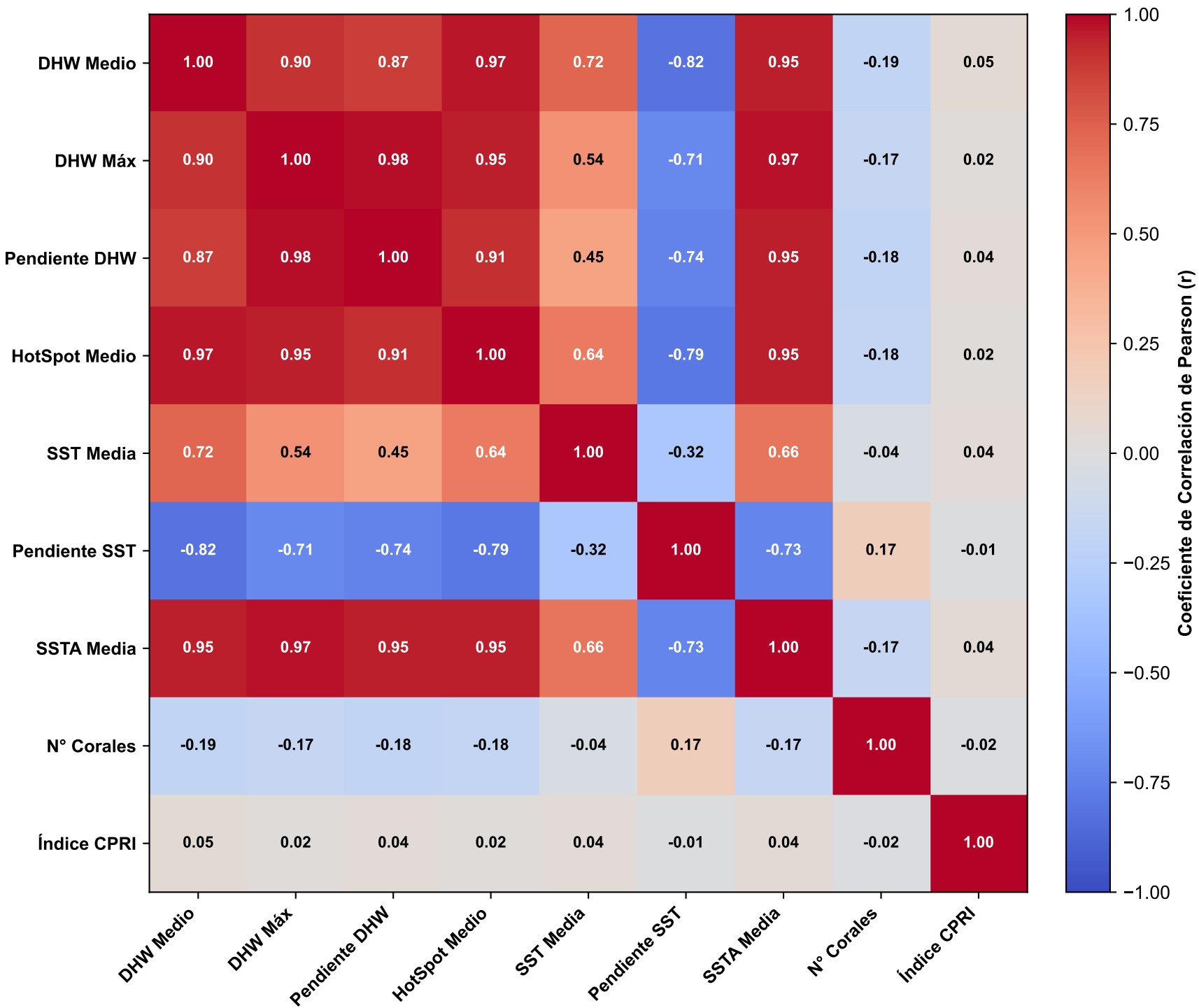
Matriz de Correlación entre Variables Oceanográficas e In Situ del SAM
