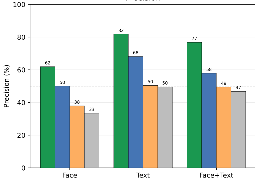
Precision
