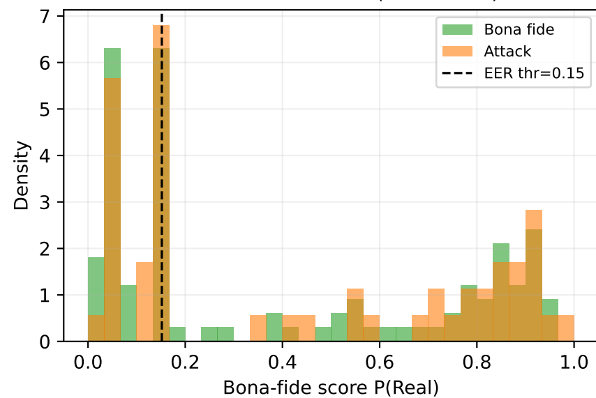
Baseline - Face Attack (AUC=0.469)
