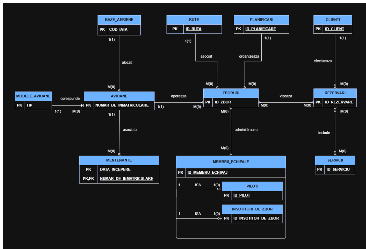
Figura 4.1. Diagrama Entitate-Relație (E/R) asociată modelului prezentat în cadrul capitolului 2
