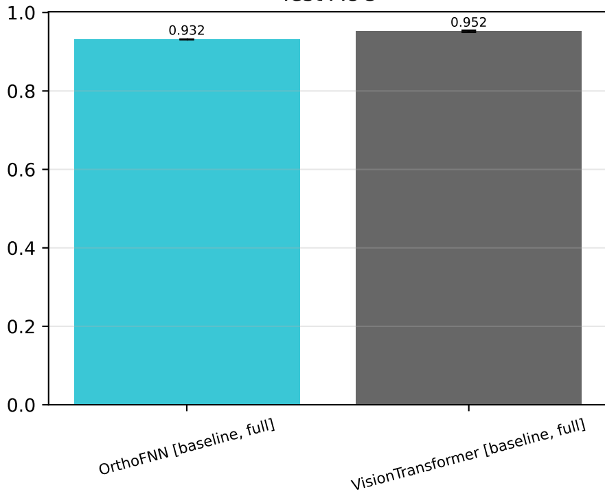
Test AUC
