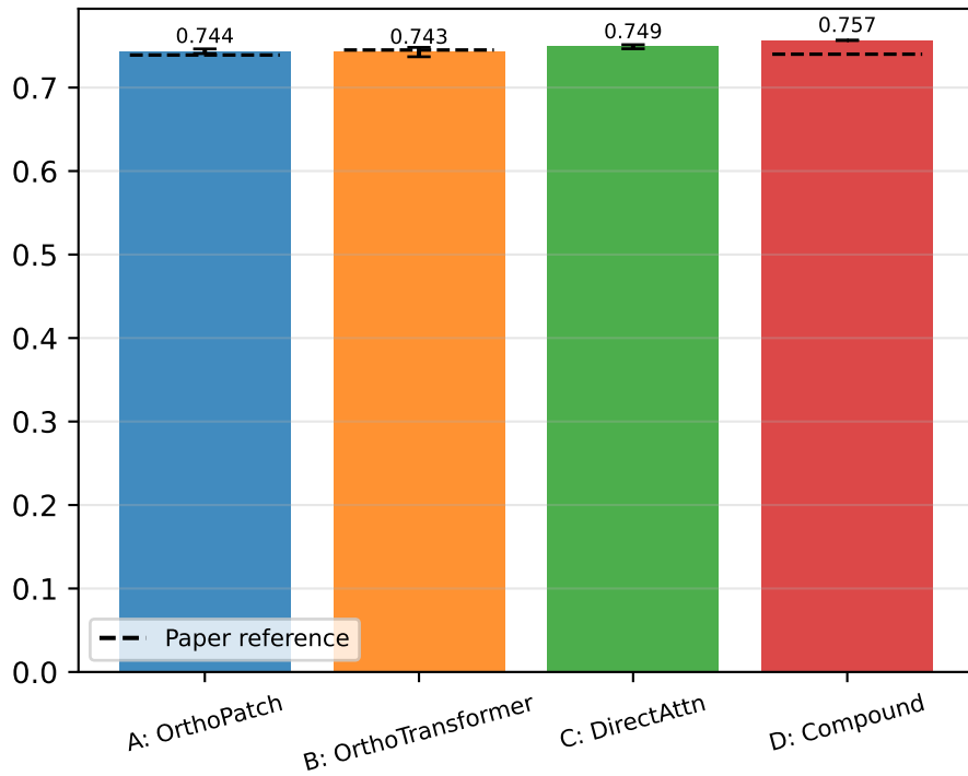
Test AUC
