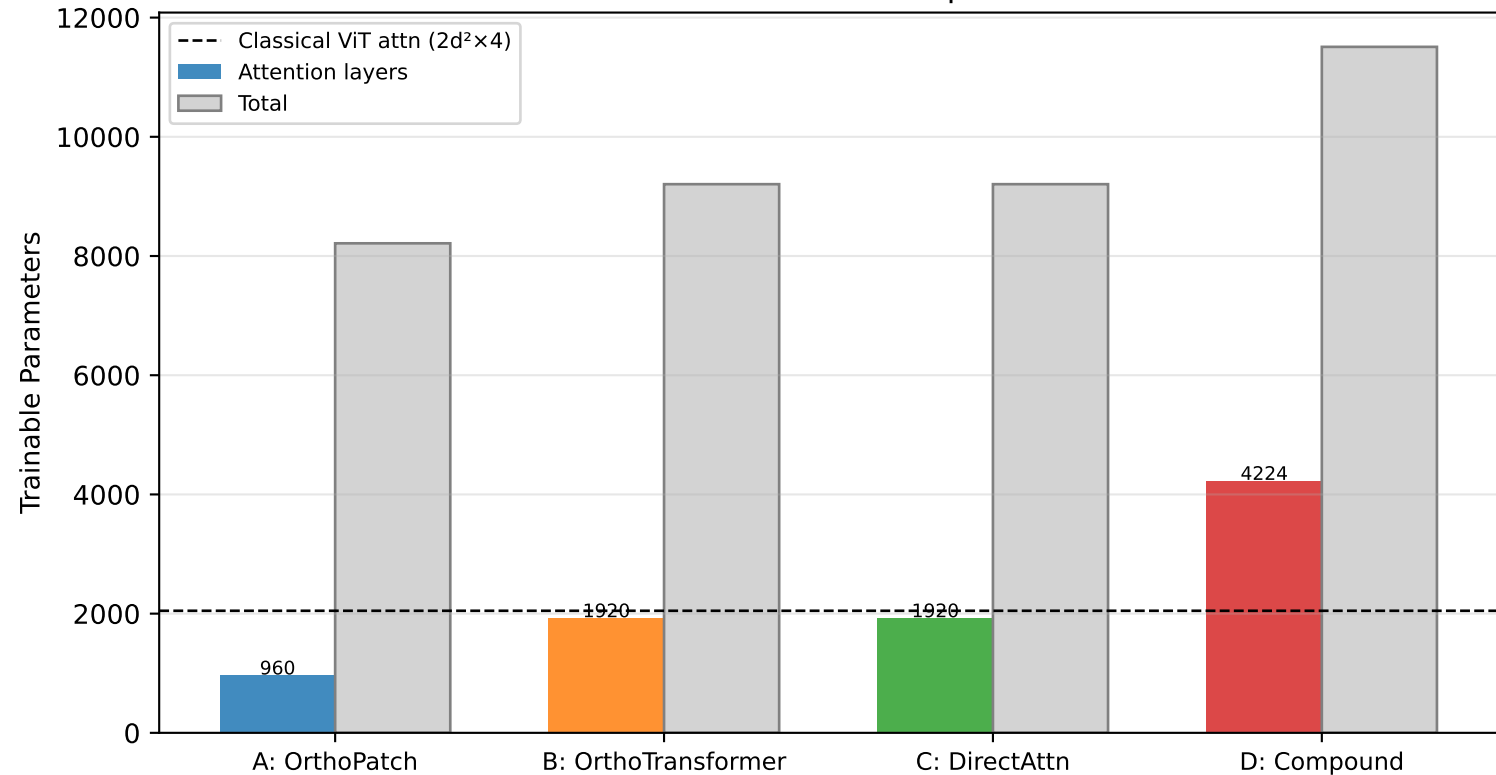
Parameter Count Comparison
