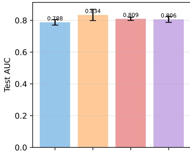
Test AUC
