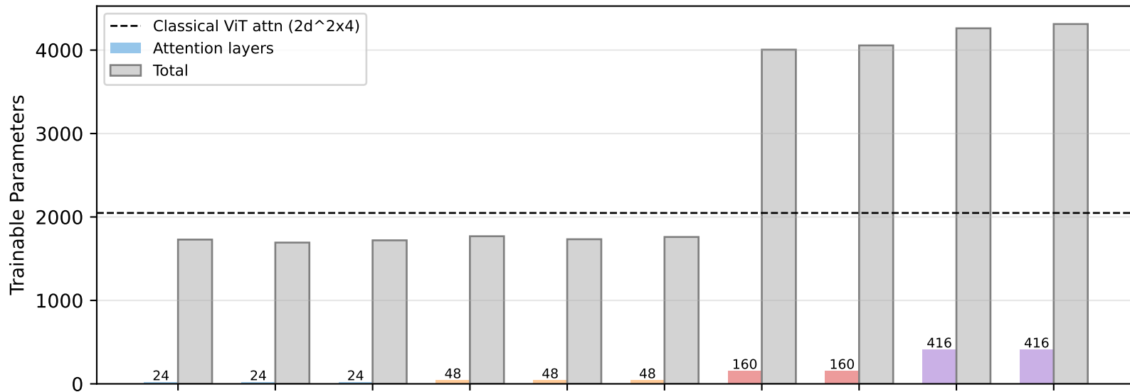
Parameter Count Comparison
