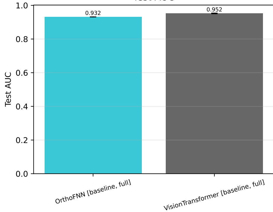
Test AUC
