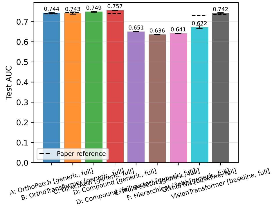
Test AUC
