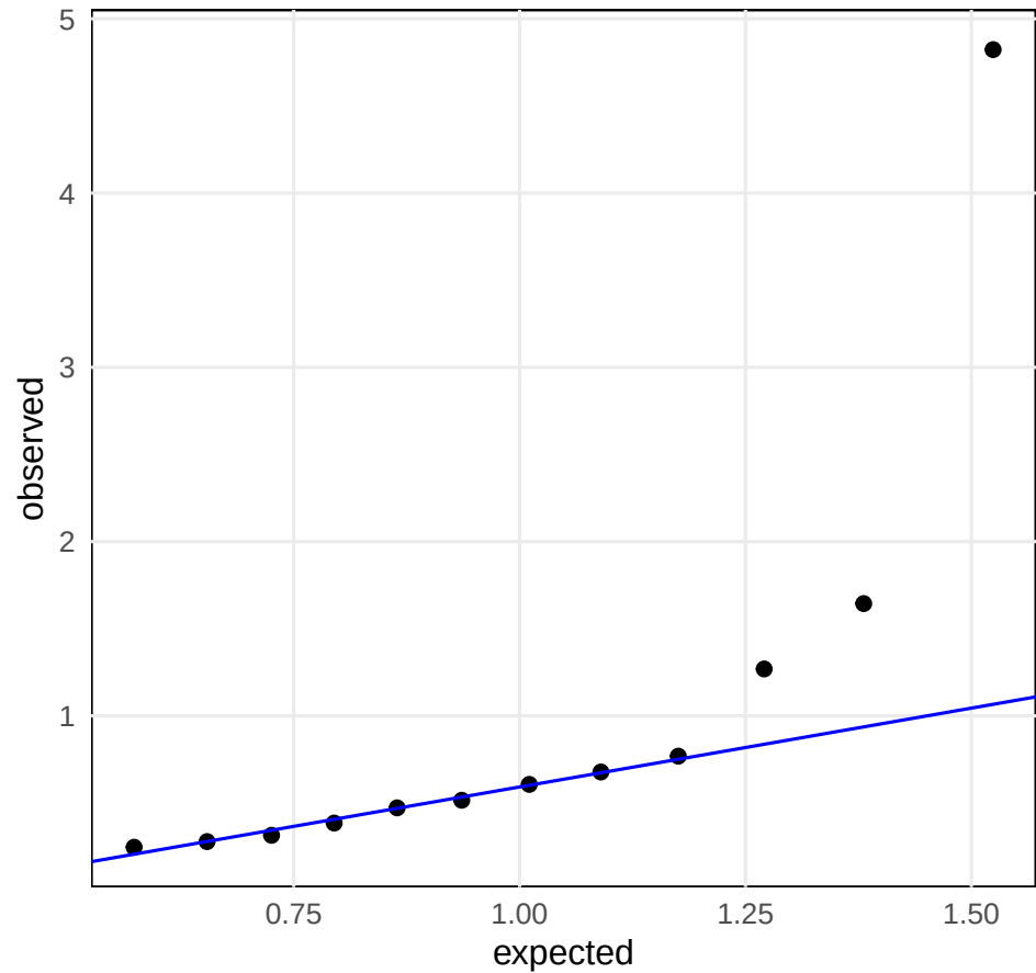
wachter qq-plot
