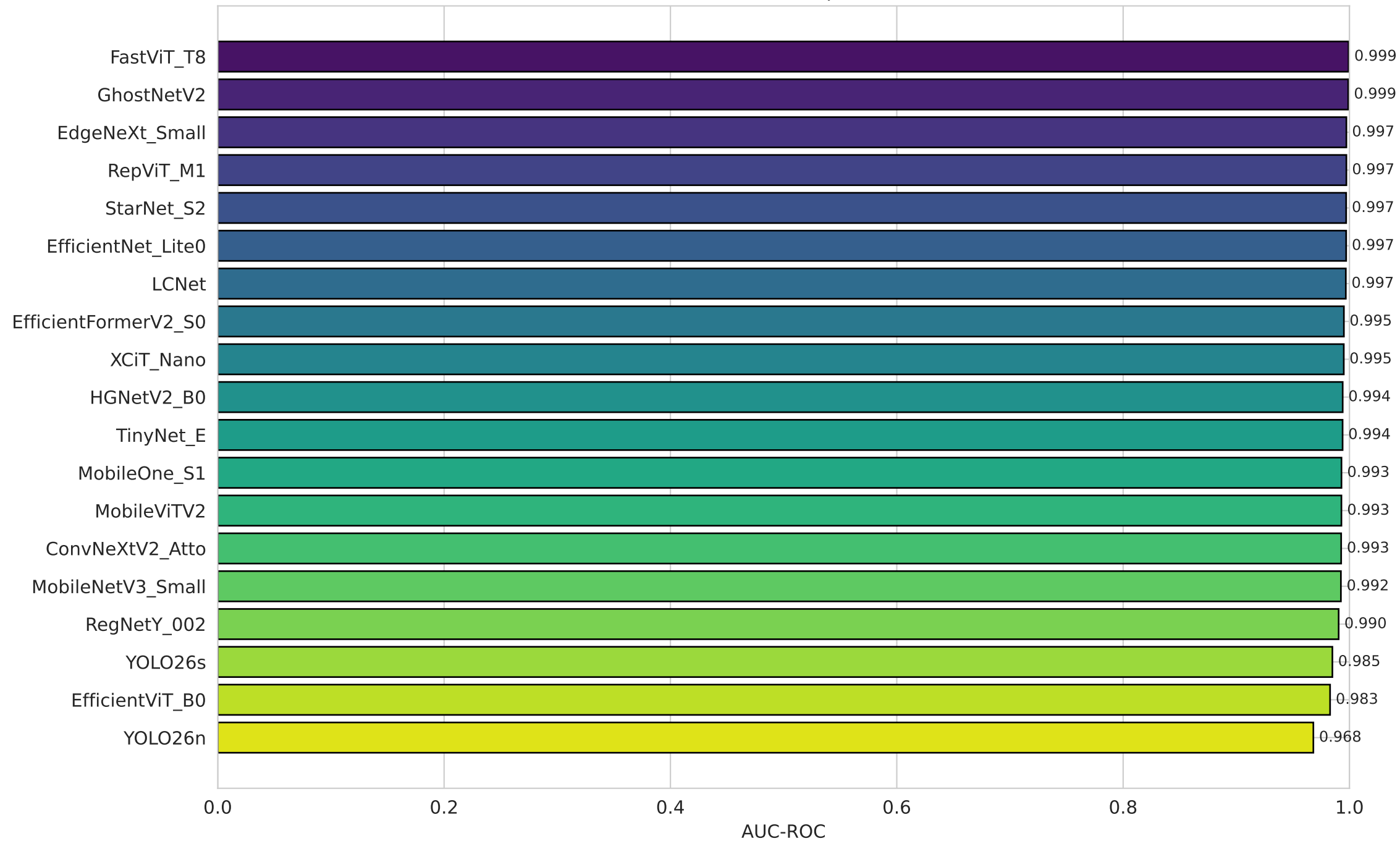
Cat Thermal — Model Comparison (AUC-ROC)
