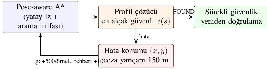
Şekil 17.1: Yatay arama ile irtifa profili arasındaki geri besleme döngüsü (plan_terrain_following)
