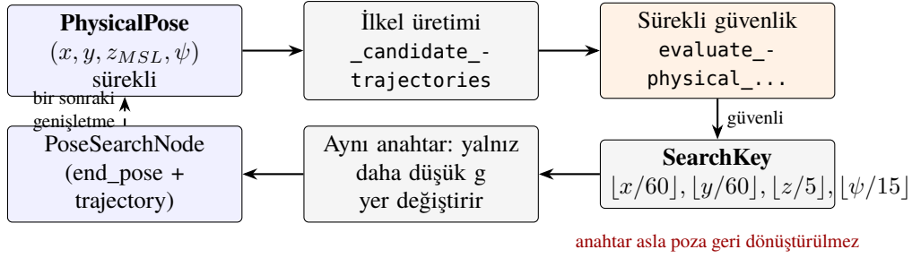
Şekil 7.1: Arama durumu (SearchKey) ile fiziksel poz ayrımı
