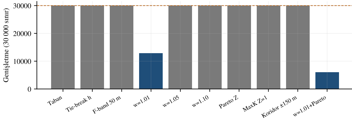
Şekil 5.1: Mission E azaltma varyantları, genişletme sayısı. Mavi: çözüm bulundu; gri: 30 000 sınırı. Veri: vertical_bottleneck_mitigation_report.md §2.
