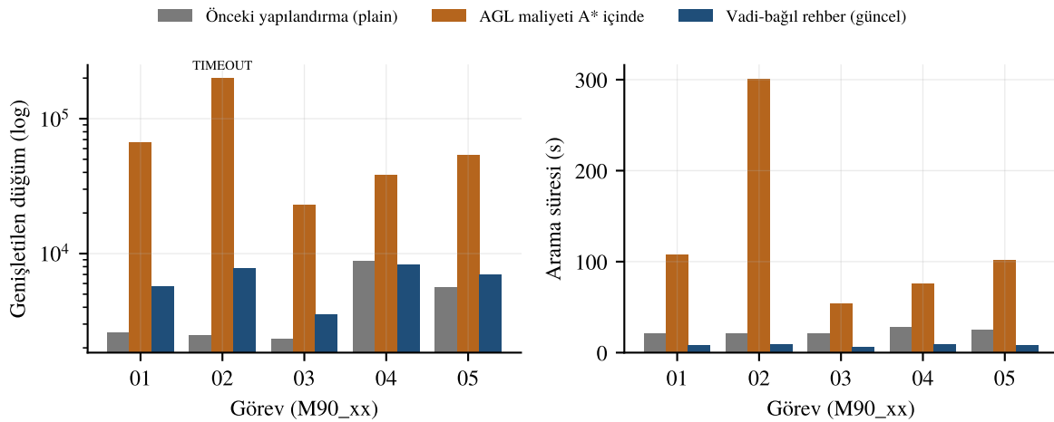
Şekil 20.1: Tablo 20.1'in grafiği. Sol: genişletme (log ölçek). Sağ: arama süresi. M90_02'nin AGL maliyetli koşusu TIMEOUT'tur, çubuk 200 001 genişletme / 301 s'yi gösterir.
