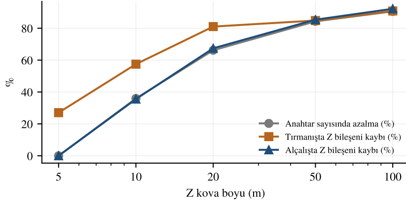
Şekil 8.1: Mission E'de 30 000 gerçek temsilcinin çevrimdışı Z yeniden kovalanması. Veri: mission_e_z_state_redundancy_diagnostic.md.
