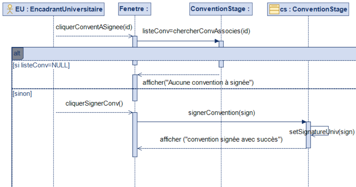
FIGURE 2.1.5 – Diagramme de séquence : Signature de la convention de stage
