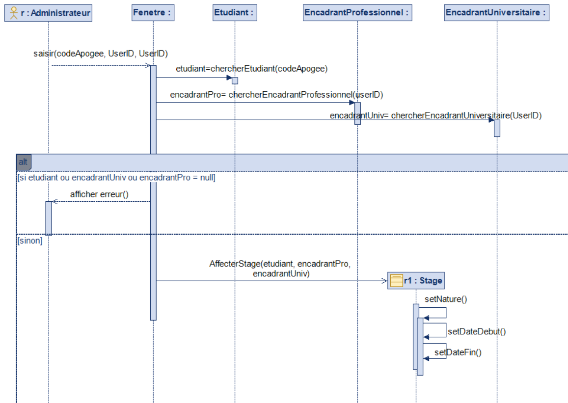
FIGURE 2.1.3 – Diagramme de séquence : Affectation des Stages
