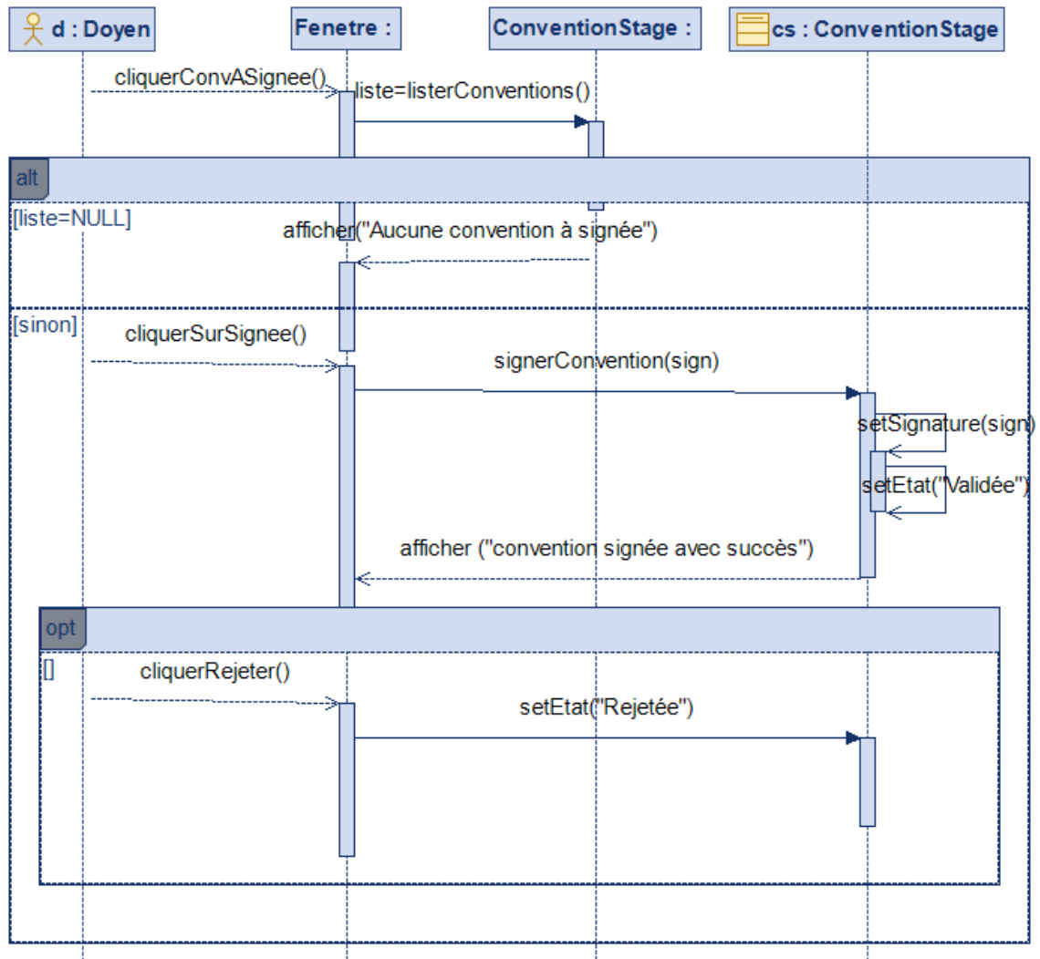
FIGURE 2.1.7 – Diagramme de séquence : Validation des conventions par le Doyen ou Vice-Doyen
