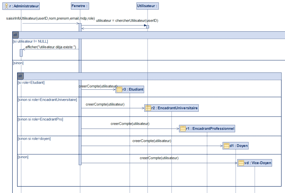
FIGURE 2.1.2 – Diagramme de séquence : Création des comptes par l'administrateur
