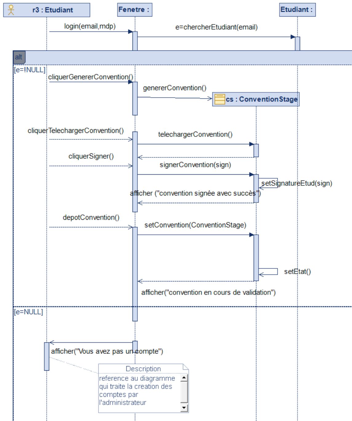
FIGURE 2.1.4 – Diagramme de séquence : Génération et dépôt de convention
