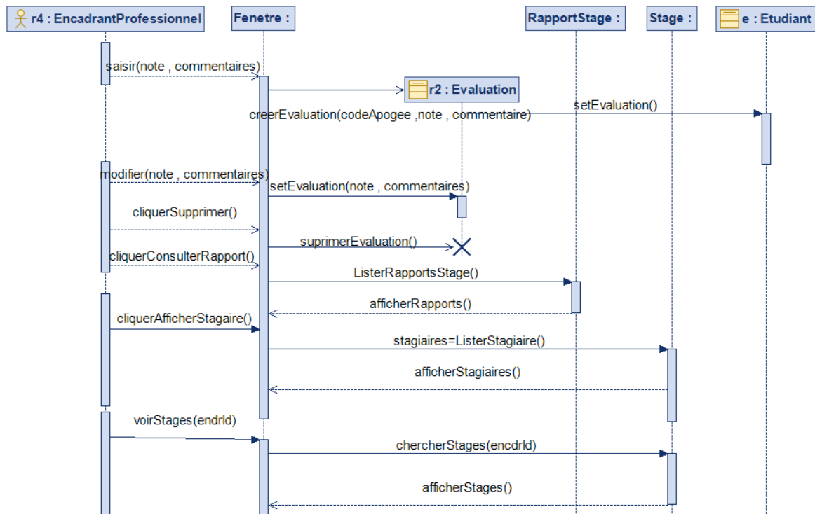
FIGURE 2.1.6 – Diagramme de séquence : Évaluation et suivi des étudiants en stage
