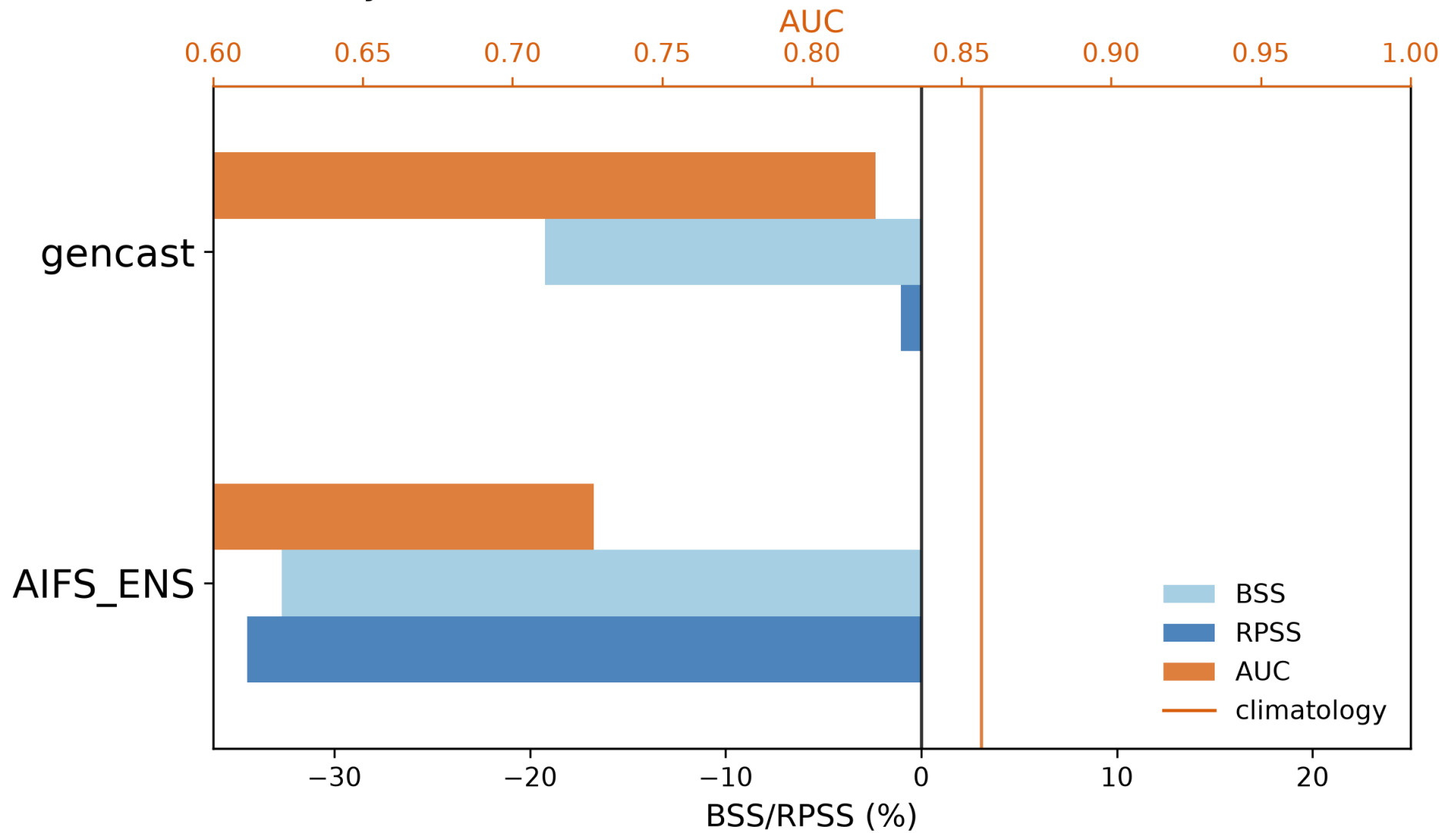
Panel Bar Bss Rpss Auc 1-15 - Days 1-15
