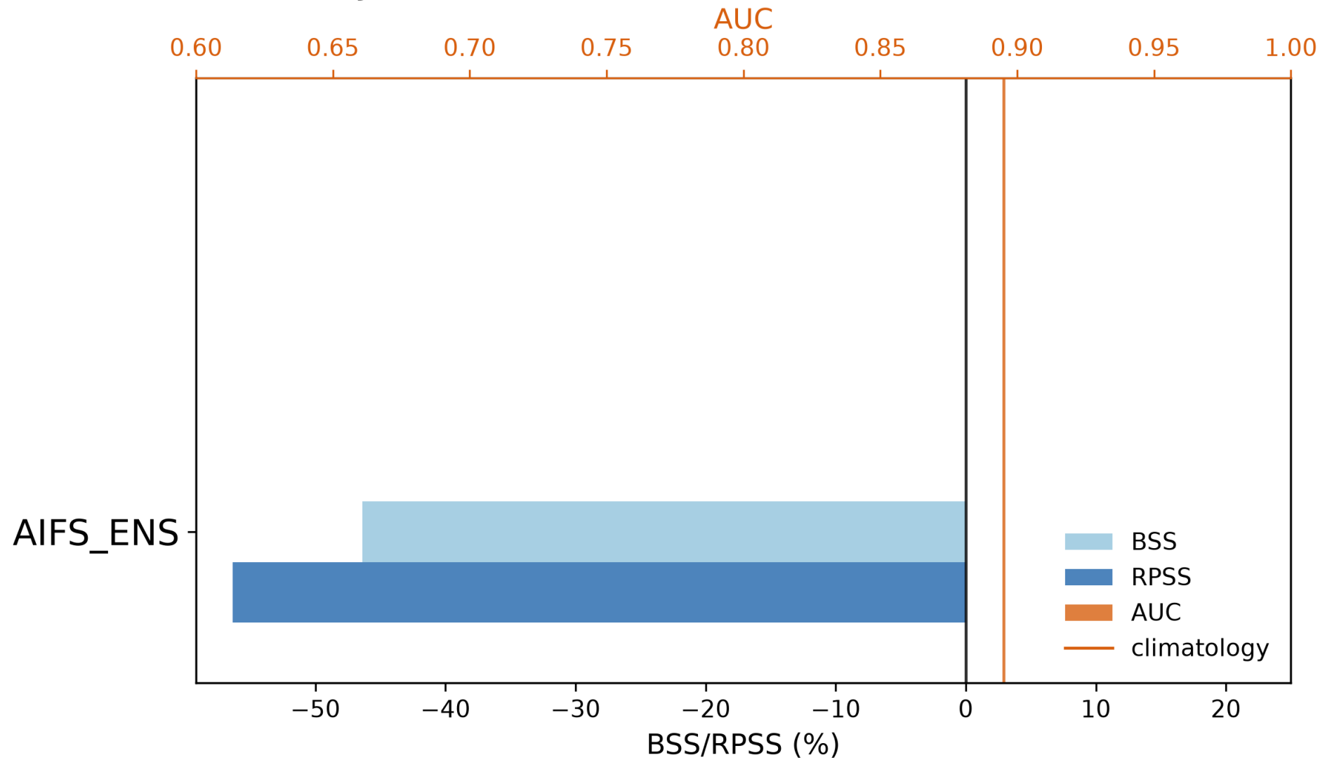
Panel Bar Bss Rpss Auc 16-30 - Days 16-30
