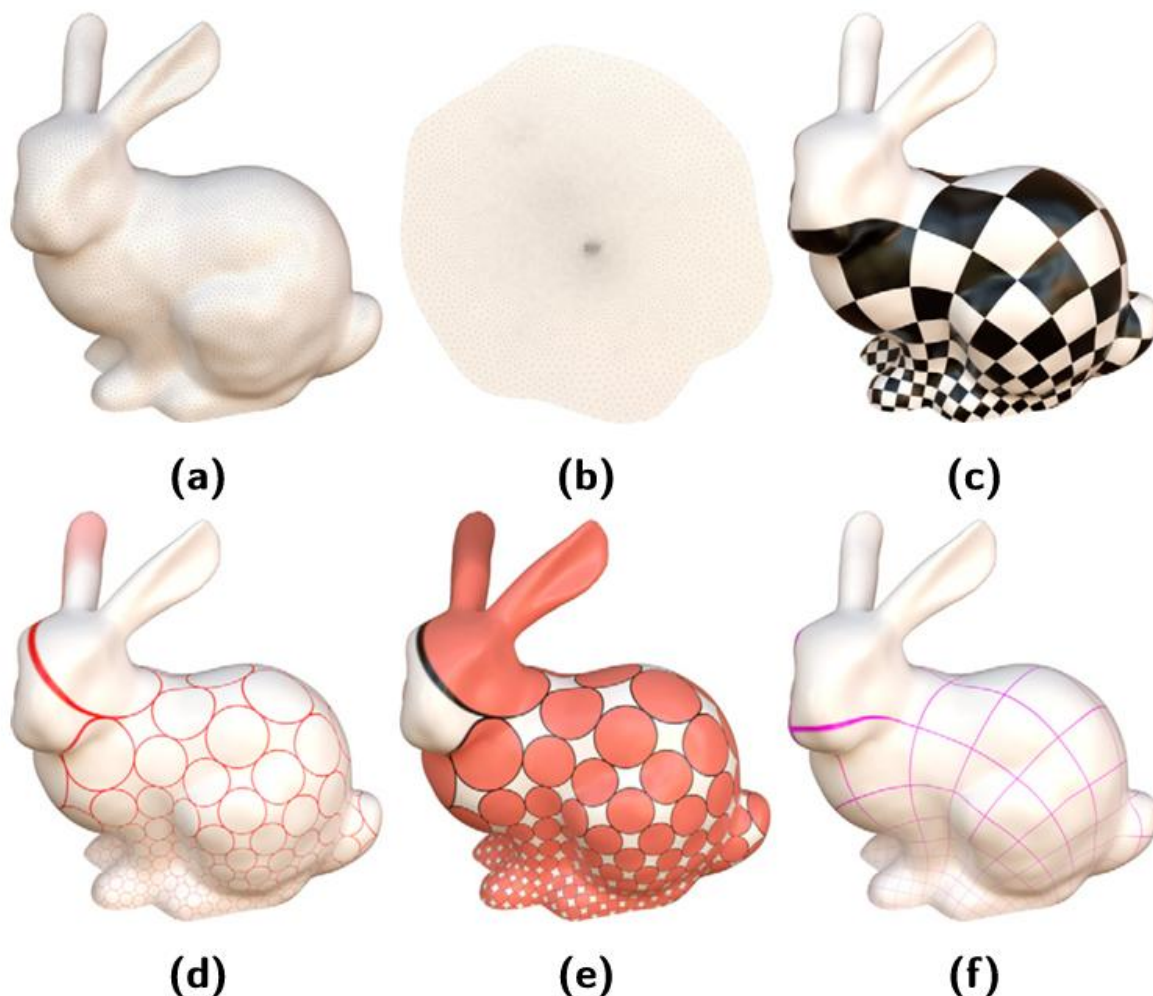
(图 31: 碟形参数化。)
