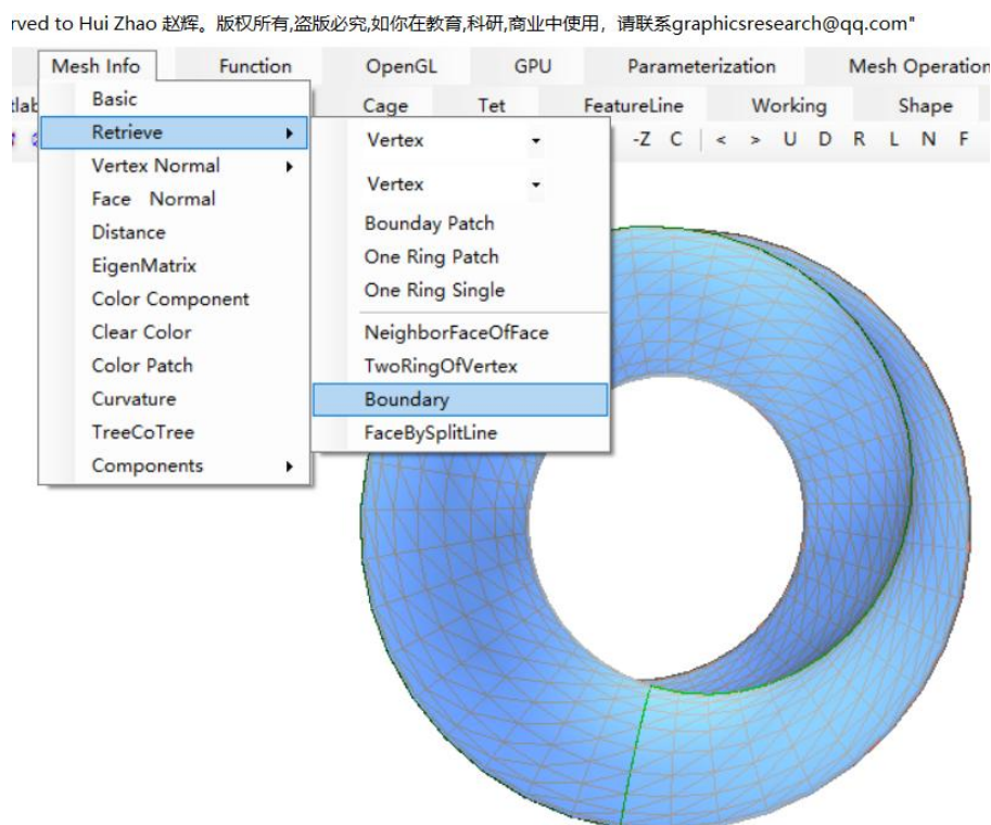
(图 4: Umbilic Torus 边界。)
