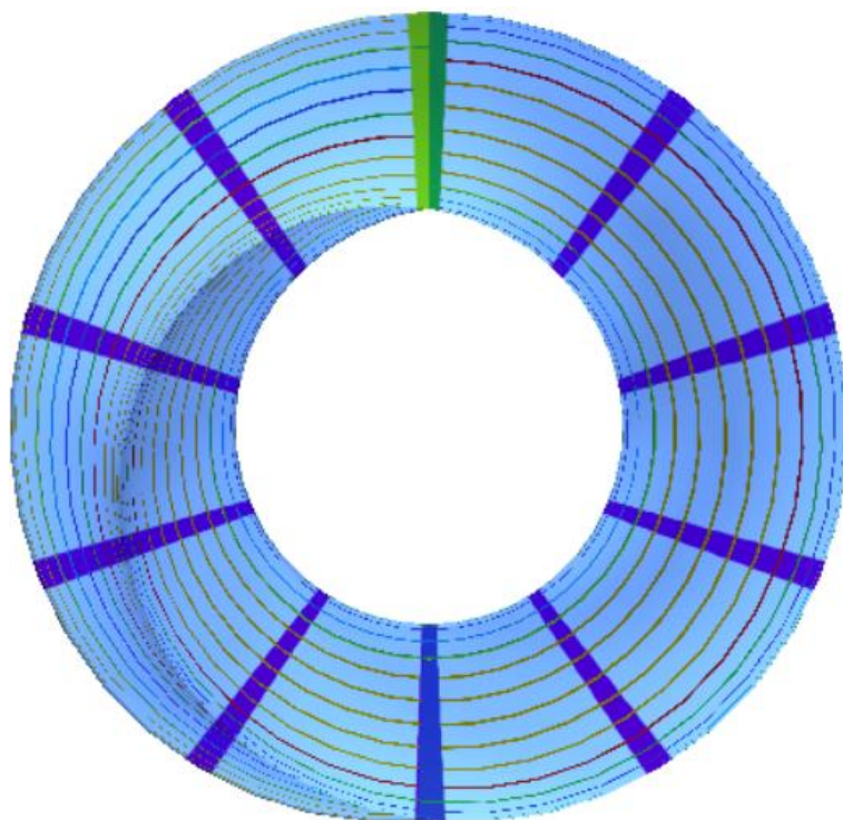
(图 7: 有错切的 Umbilic Torus。)
