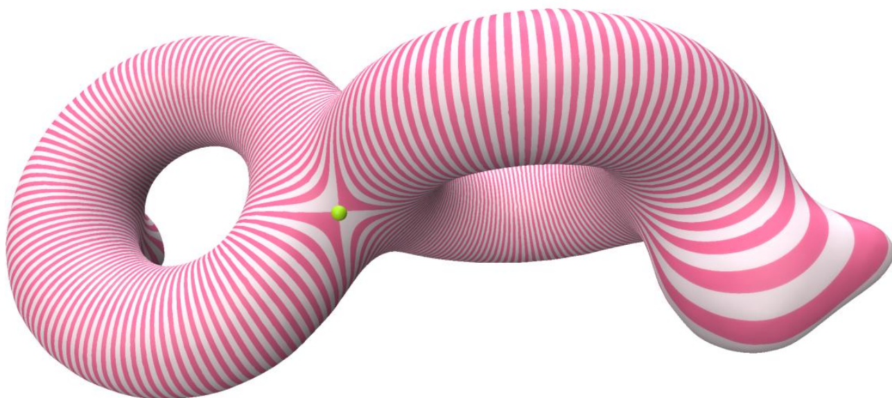
(图 26: 调和叶状结构, 赵辉用 Geometric 作图。)
