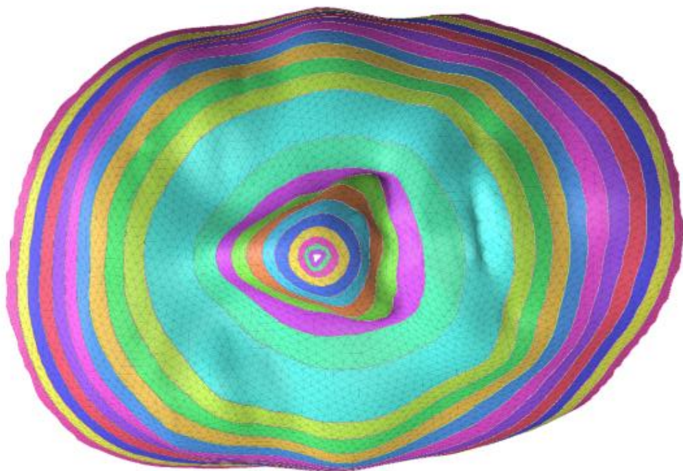
(图 20: 有边界曲面上的调和叶状结构, Geometric 作图。)
