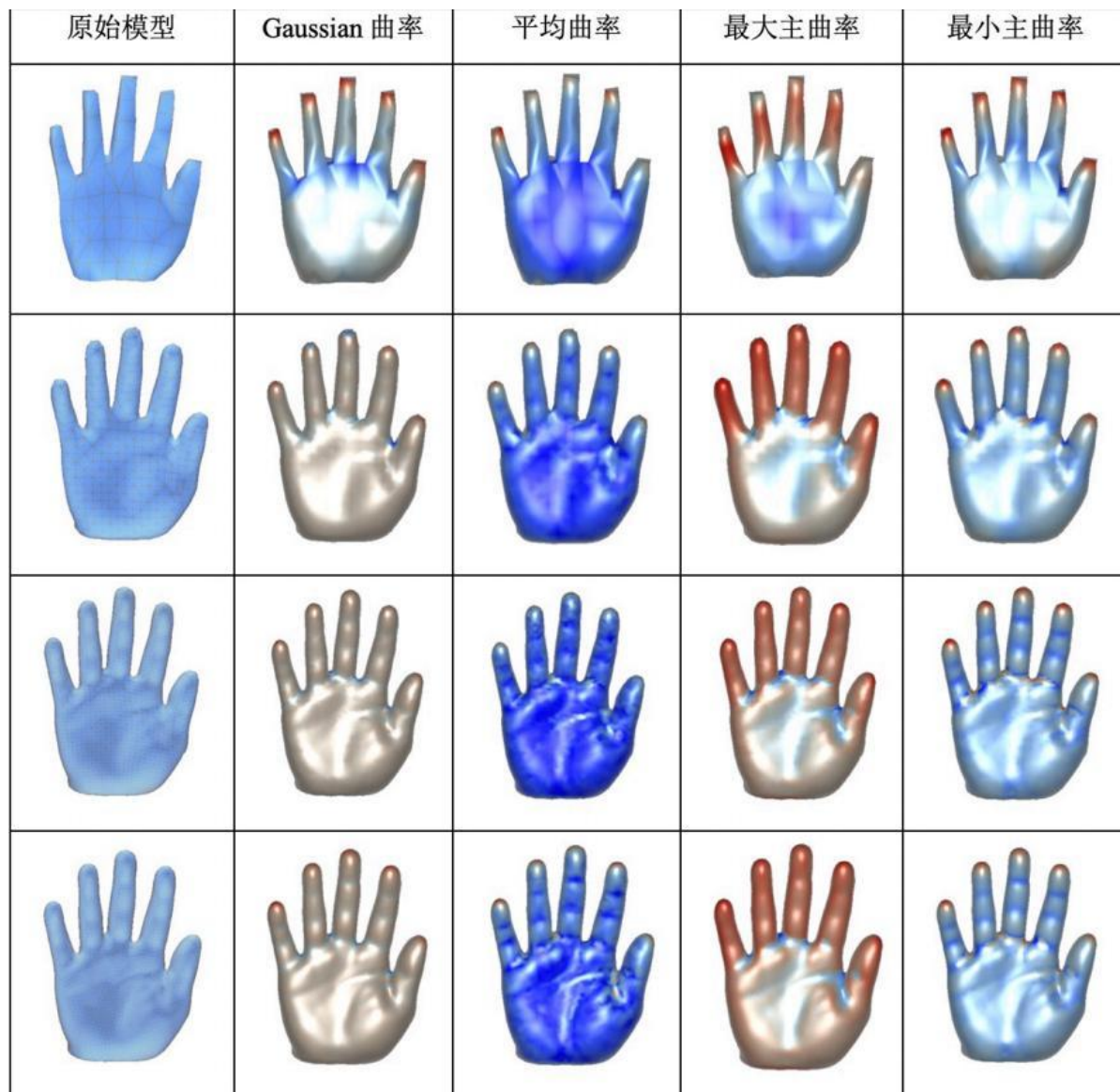
(图 8: 各种曲率, 不同的颜色表示不同数值的曲率, meshDGP 作图。) (Figure 8: Several kinds of curvatures, curvature numerical value are colored.)
