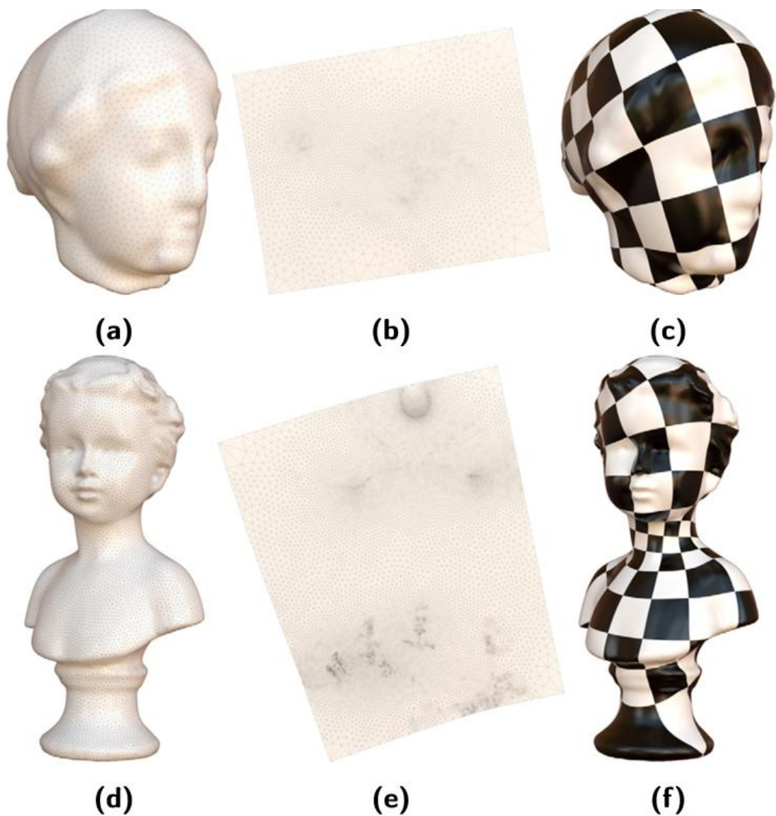
(图 45： 平直度量。) (Figure 45: Flat metric and parameterization .)
