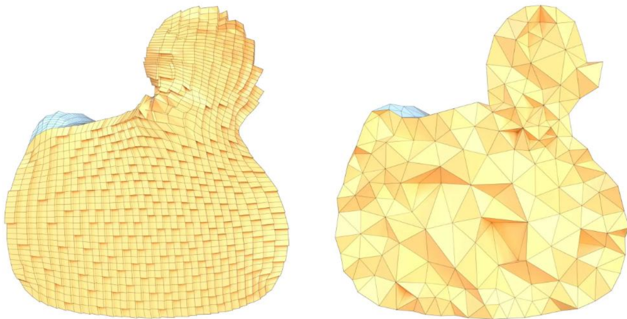
(图 42：结构化和非结构化网格，原创几何拓扑代码平台 Geometric 作图。)
