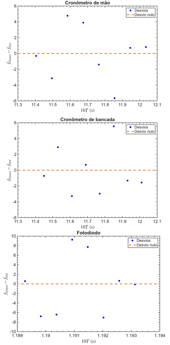
Figura 6: Desvios clculados para experimento com fotodiodo
