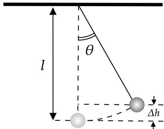
Figura 1: Esquemática de um pêndulo simples
