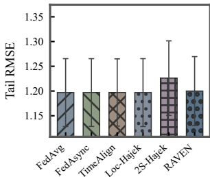
(d) U-Air, Tail RMSE
