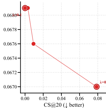
TRIER-L
