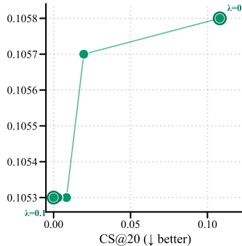
TRIER-C
