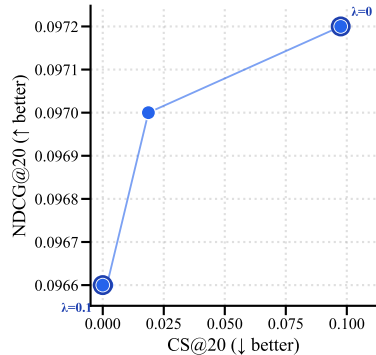
TRIER
