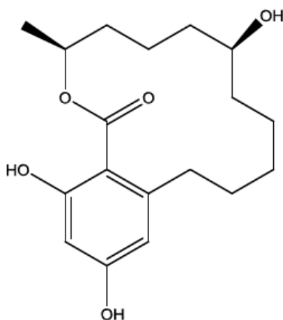
Figure 2-7 — (β)-Zearalanol (β-ZAL), C 18 H 26 O 5 ; MW : 322.396 Da; P kw : - 3.86
