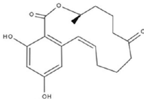
Figure 2-5 — cis -Zearalenone ( cis -ZEN); C 18 H 22 O 5 , MW : 318.36 Da;
