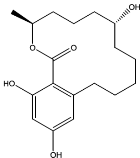
Figure 2-6 — (α)-Zearalanol (α-ZAL), C 18 H 26 O 5 MW : 322.396 Da; P kw : - 3.86
