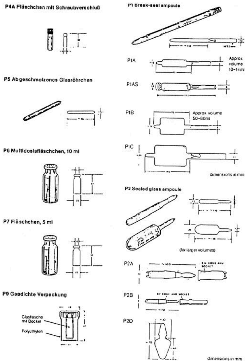
Figure 51 — Various ampoules and vials used by manufacturers of radioactive sources, for example the P6 multidose vial for solutions or P1A for radioactive gases (Fläschchen mit Schraubverschluß ⇒ vial with screw cap, Abgeschmolzenes Glasröhrchen ⇒ sealed glass tube, Multidosisfläschchen ⇒ multidose glass vial, Fläschchen ⇒ vial, Gasdichte Verpackung ⇒ gas tight packaging, Glasflasche mit Deckel ⇒ capped glass vial). Reproduced from [6].
