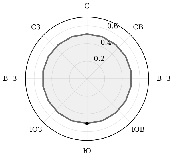
(б) Термический компонент (0.51)
