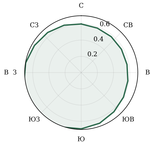
(в) Совокупный
