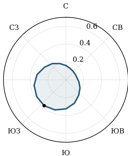
(а) Ветровой компонент
