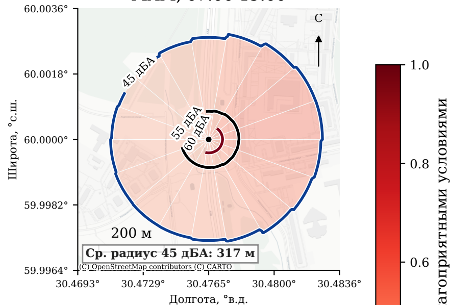
Статический расчёт МГСУ без C_{\text{met}}
