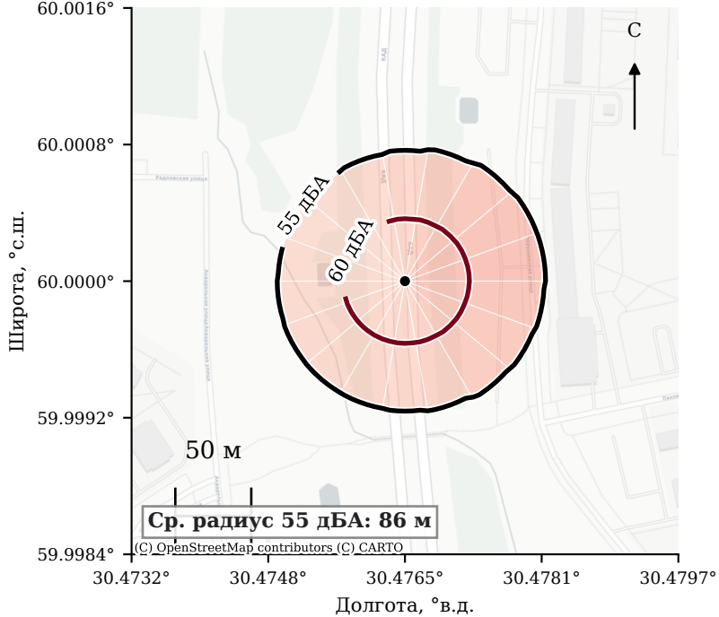
Статический расчёт МГСУ без C_{\text{met}}
