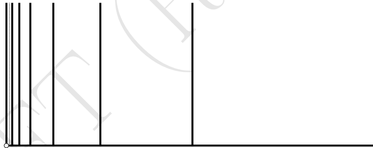
Figura 4.4: Esboço do espaço pente. Note que a origem (0, 0) não pertence a este espaço.
