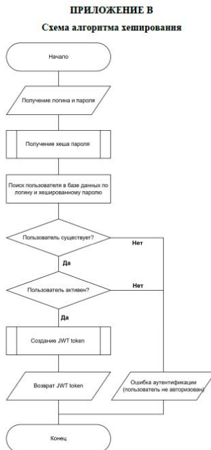
Рисунок В.1 – Схема алгоритма хеширования
