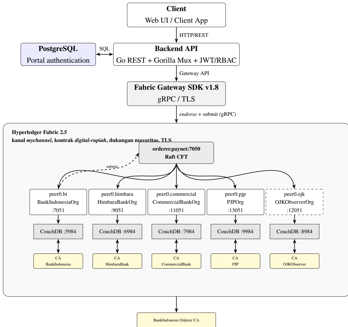
Gambar 3.22. Arsitektur sistem Rupiah Digital: lapisan client , backend API (Go REST + JWT/RBAC), basis data PostgreSQL luring, Fabric Gateway SDK , serta jaringan Hyperledger Fabric 2.5 dengan lima organisasi peer , CouchDB, CA per organisasi, dan orderer Raft
