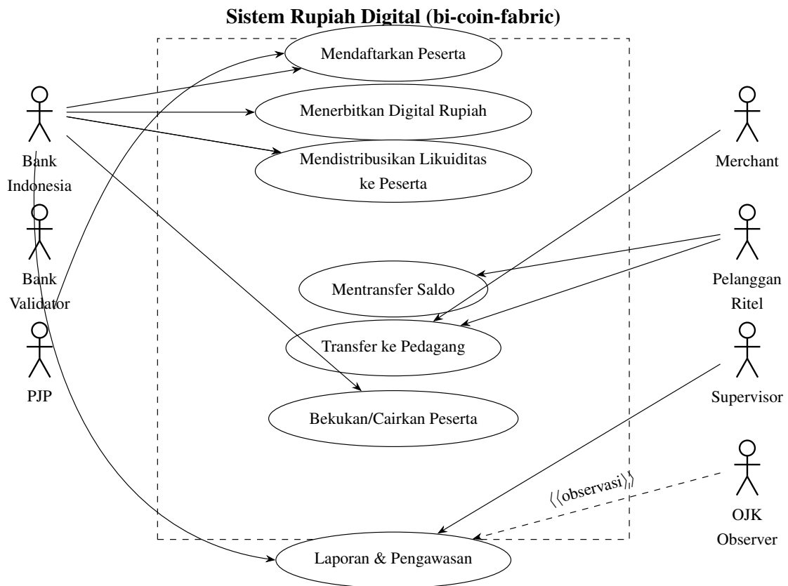
Gambar 3.24. Diagram use case keseluruhan sistem Rupiah Digital
