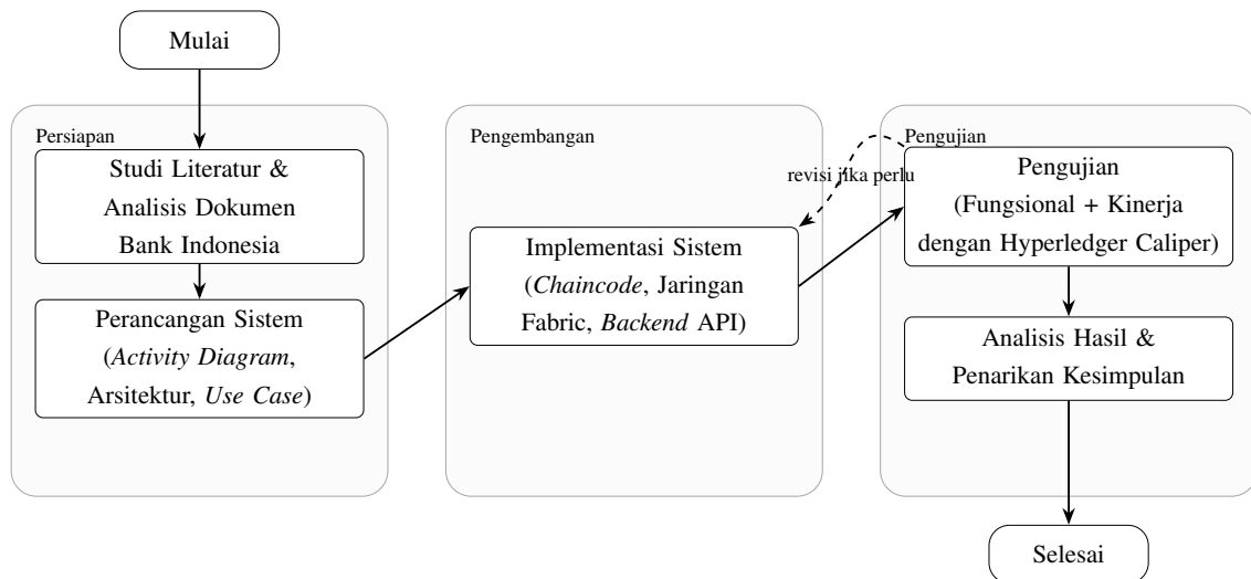
Gambar 3.27. Alur pelaksanaan tugas akhir: dari studi literatur hingga penarikan kesimpulan, dengan umpan balik iteratif antara implementasi dan pengujian
