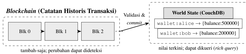
Gambar 2.10. Dualitas komponen ledger Hyperledger Fabric: blockchain sebagai catatan transaksi historis tambah-saja yang perubahannya retrospektifnya dapat dideteksi, dan world state sebagai representasi status terkini pada CouchDB
