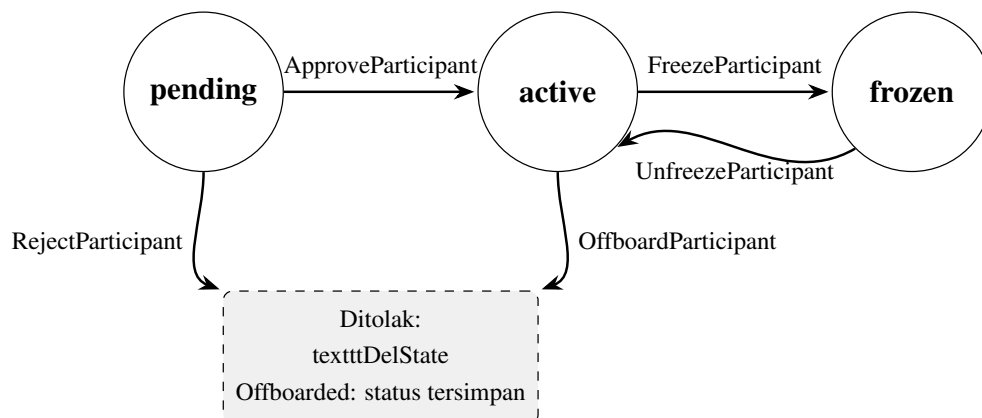
Gambar 4.31. Siklus hidup peserta pada chaincode : dari pending (menunggu persetujuan) menjadi active , kemudian dapat dibekukan ( frozen ) dan dicairkan kembali. Penolakan menghapus peserta yang masih pending , sedangkan OffboardParticipant menyimpan status offboarded , membekukan dompet terkait, dan mensyaratkan saldo agregat nol.
