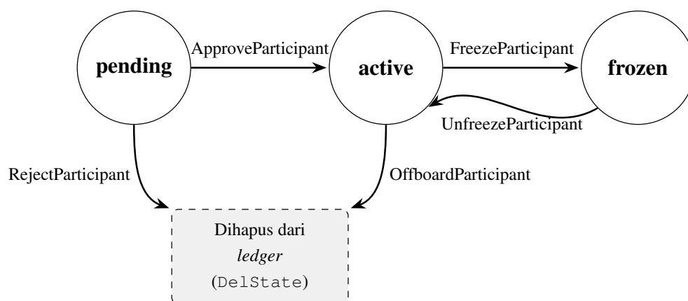
Gambar 4.35. Siklus hidup peserta pada chaincode : dari pending (menunggu persetujuan) menjadi active , kemudian dapat dibekukan ( frozen ) dan dicairkan kembali. Penolakan ( RejectParticipant ) maupun pelepasan keanggotaan ( OffboardParticipant ) menghapus rekaman peserta dari ledger ( DelState ), bukan menyimpannya sebagai status
