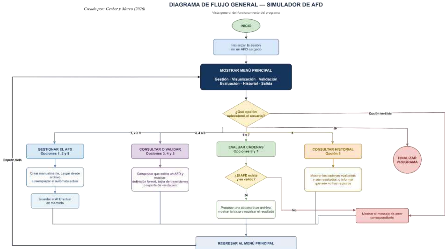
Figura 1. Diagrama de flujo general del programa para la fase 1
