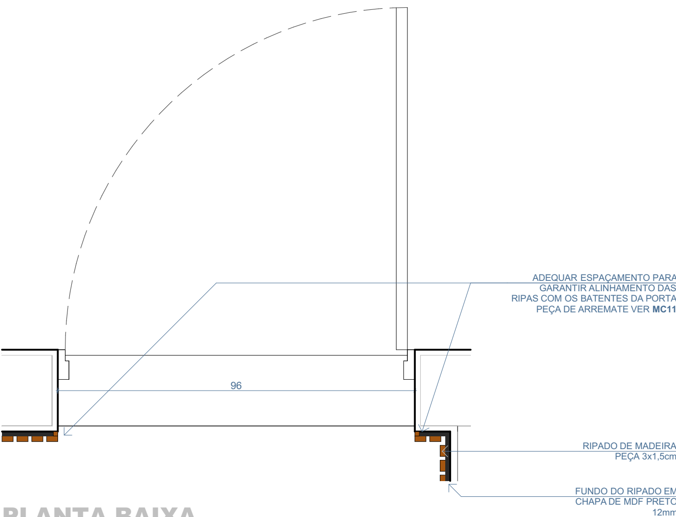
PLANTA BAIXA
