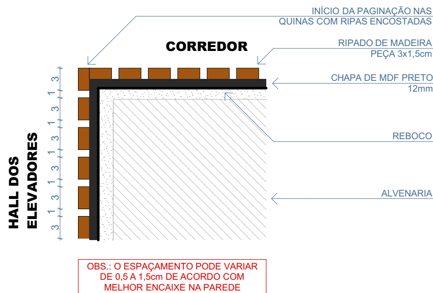
PLANTA BAIXA
