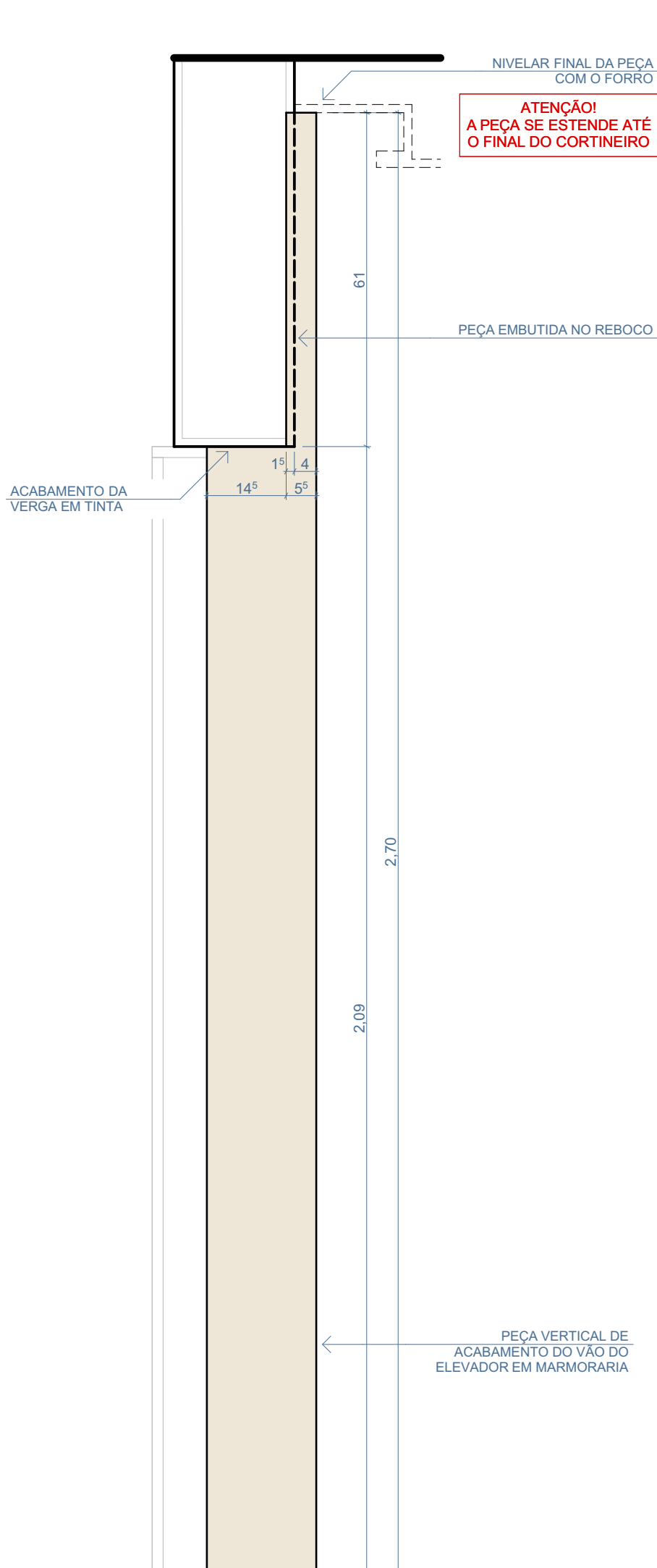
CORTE
