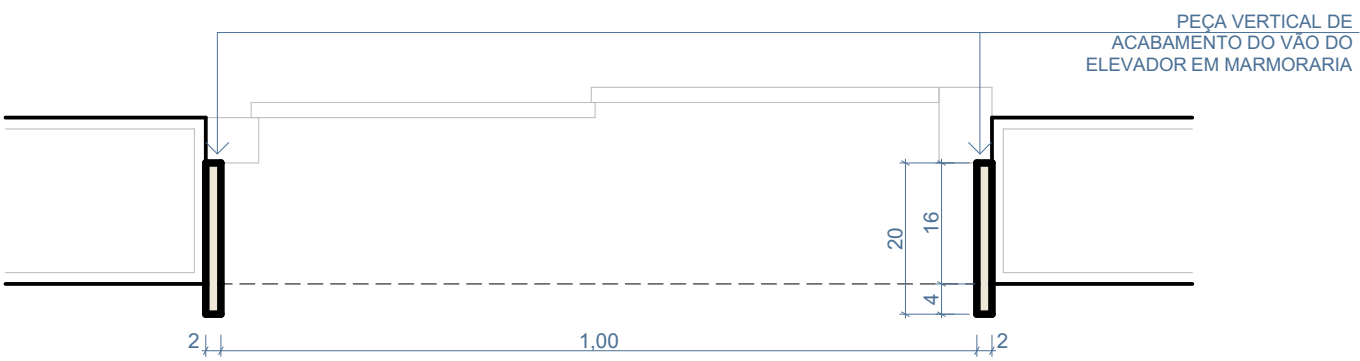
PLANTA BAIXA
