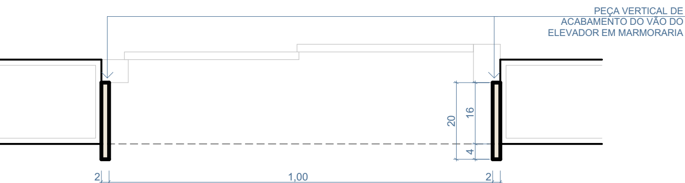
PLANTA BAIXA
