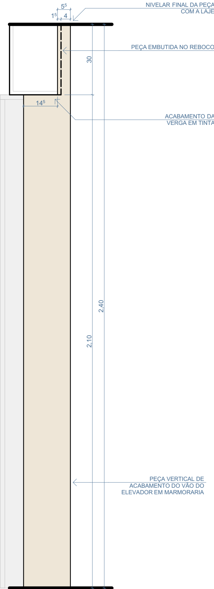
CORTE
