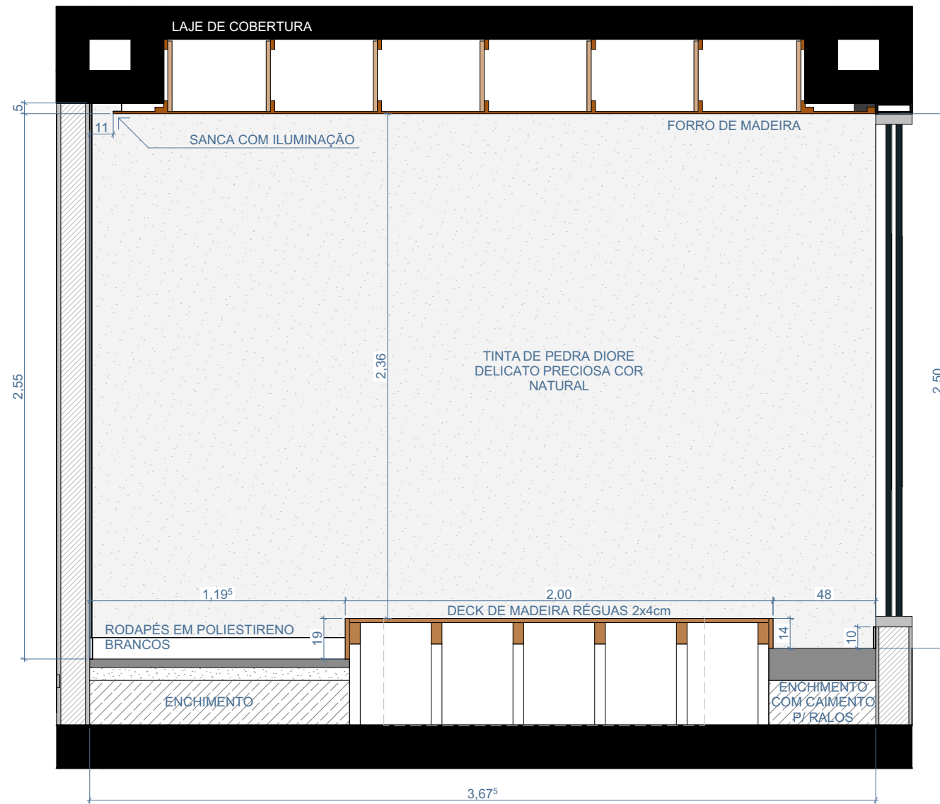
04 ESCALA 1:25
