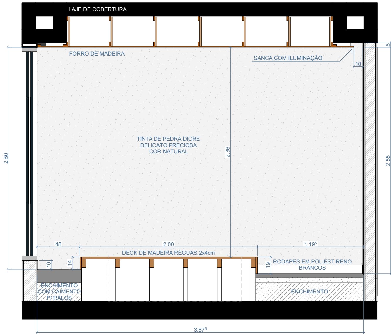
02 ESCALA 1:25
