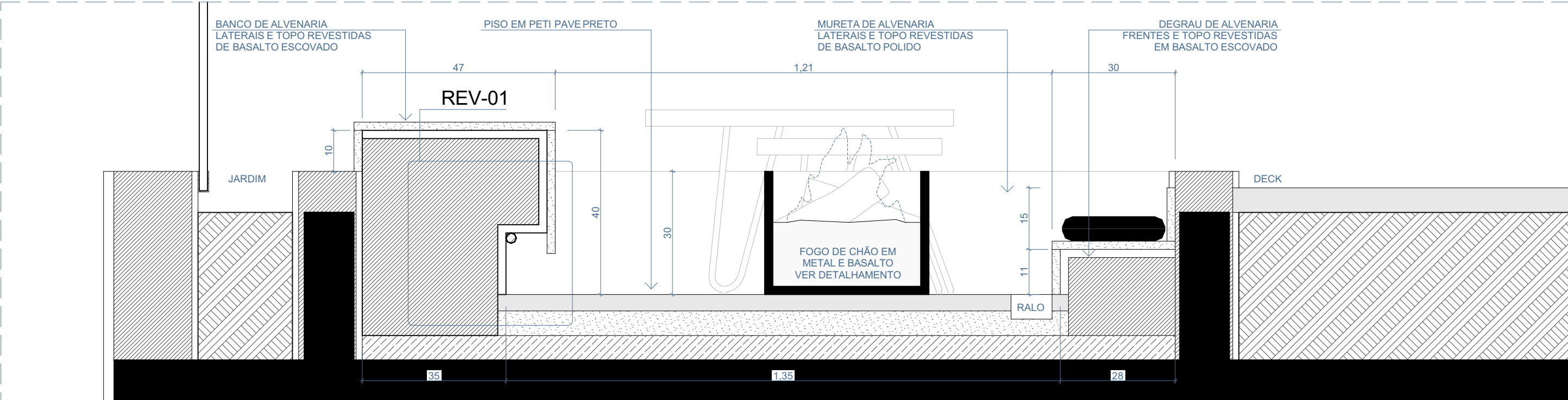
CORTE AA ESCALA 1:10
