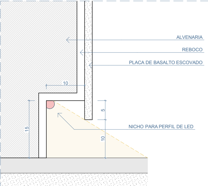
DETALHE REV-01 ESCALA 1:5
