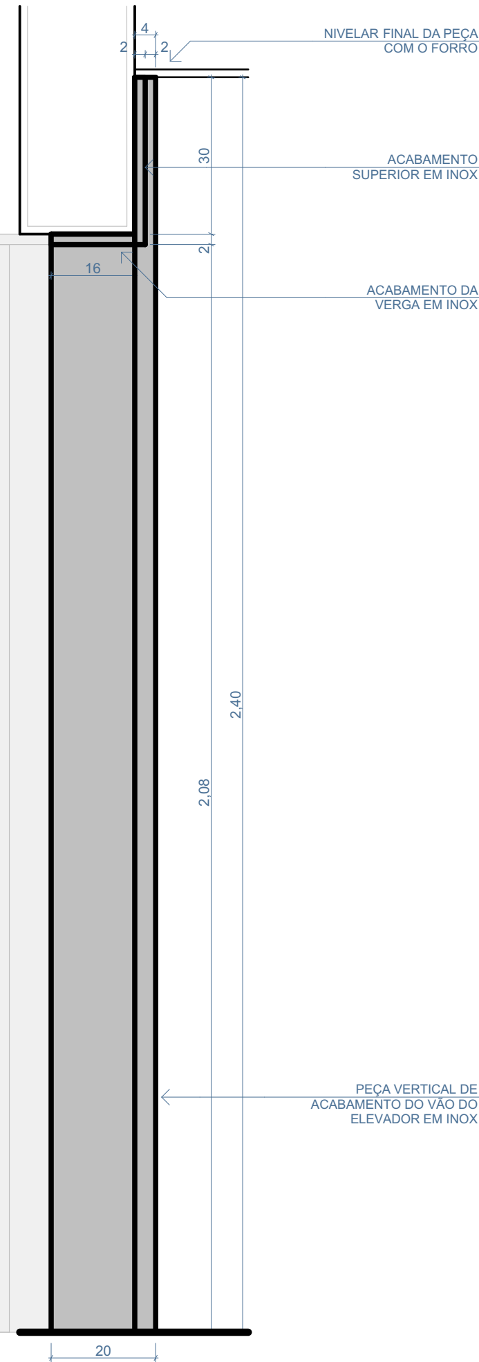
CORTE
