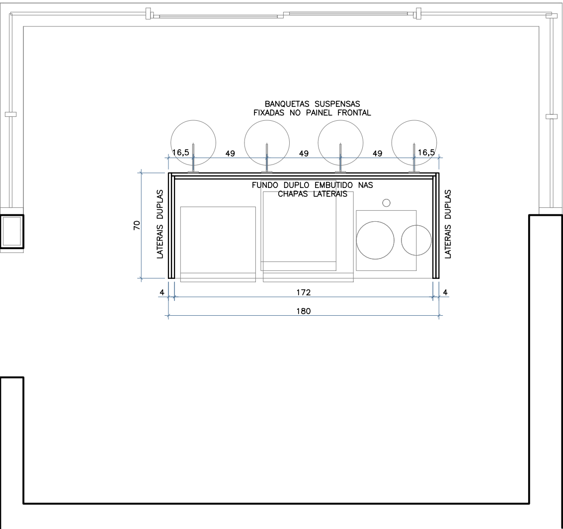
PLANTA BAIXA
