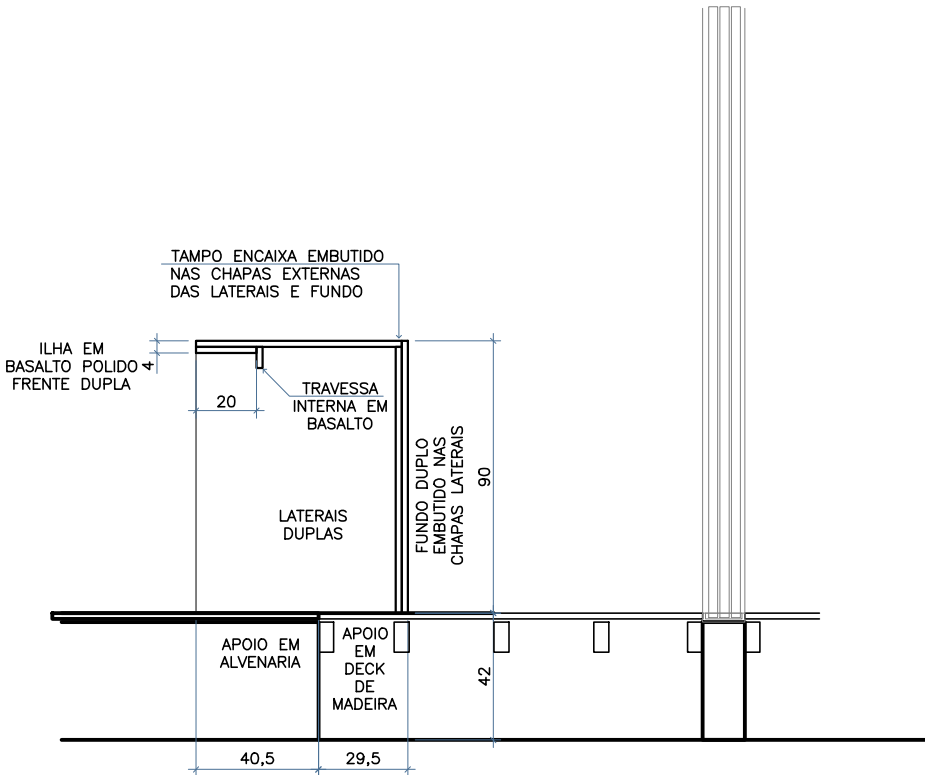
CORTE
