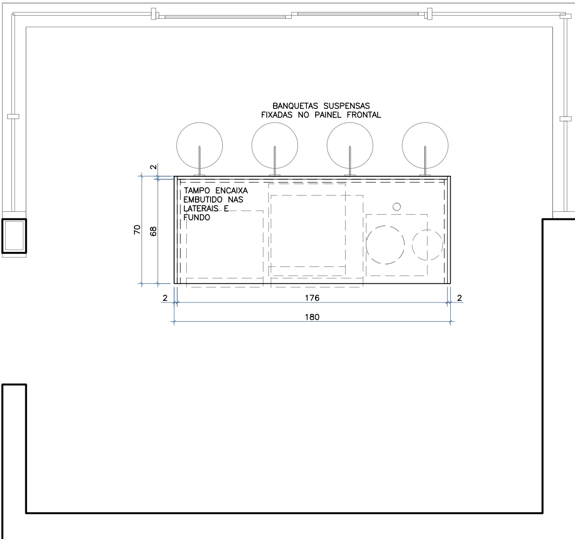
VISTA SUPERIOR
