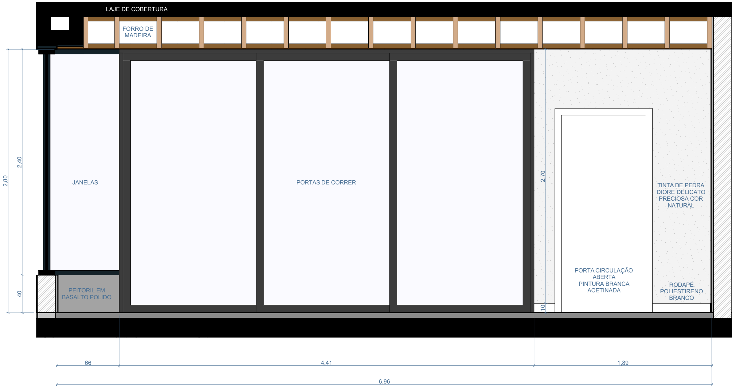
01 ESCALA 1:25
