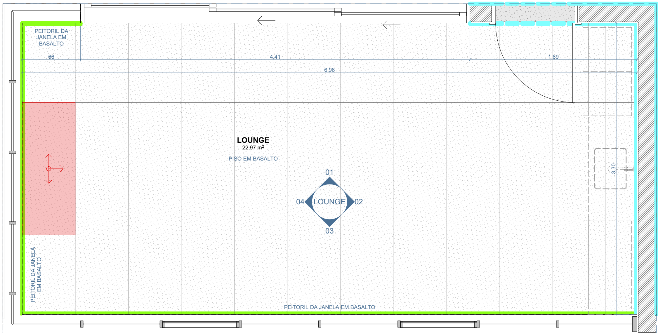
PLANTA BAIXA - LOUNGE ESCALA 1:25
