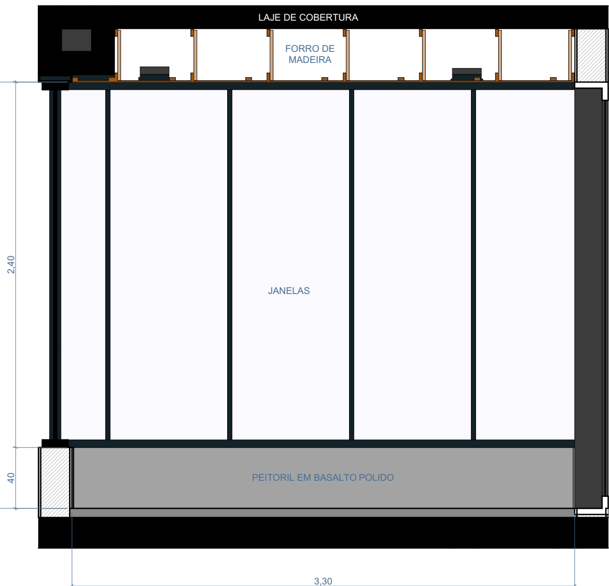
04 ESCALA 1:25
