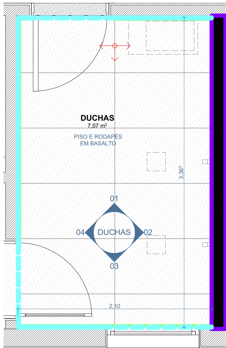
PLANTA BAIXA ESCALA 1:25
